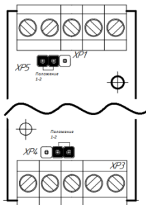
Рисунок 3 – Положение переключек
