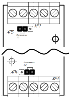
Рисунок 3 – Положение перемычек
