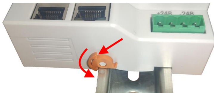
Рисунок 3-3 Фиксация интерфейсного модуля
