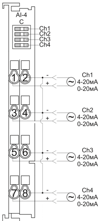
Рисунок 1 – Схема подключения модуля МАС9-4-АI-С
