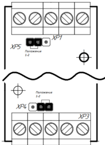
Рисунок 3 – Положение перемычек
