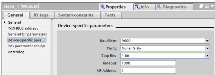
Рисунок 6 – Настройки связи Modbus RTU
