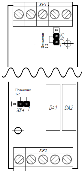
Рисунок 2 – Положение переключателей
