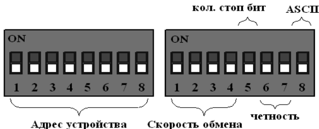
Рисунок 2 – Набор переключателей (все переключатели выключены)
