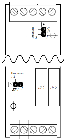
Рисунок 3 – Положение перемычек
