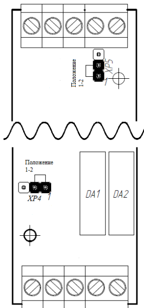
Рисунок 3 – Положение перемычек
